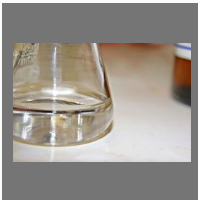
N- Hexane
