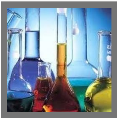
N-Propanol
